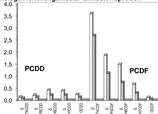
Homologenverteilungsmuster Emissionsproben
